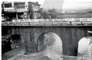
圖25 1996年以前，呈甘橋橋梁的圓拱結構。酒瓶狀欄杆已拆除，改成水平混凝土護欄，圖片來源：黃承令計劃主持，《新竹縣定古蹟關西東安橋及歷史建築芎林呈甘橋修復再利用計畫》，頁6-12。
