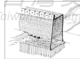
圖16 原臺北府城城牆下水洞（水關）採直樑架設結構示意圖，圖片來源：李乾朗，《臺北府城牆及礮臺基座遺址研究》，臺北市：臺北市府捷運工程局委託，1995.3，頁73。
