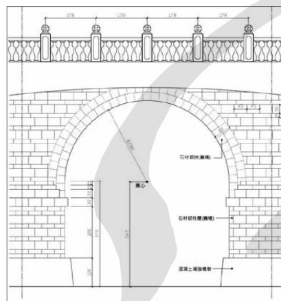
圖26 呈甘橋結構測繪圖，圖片來源：黃承令計劃主持，《新竹縣定古蹟關西東安橋及歷史建築芎林呈甘橋修復再利用計畫》，頁6-12。
