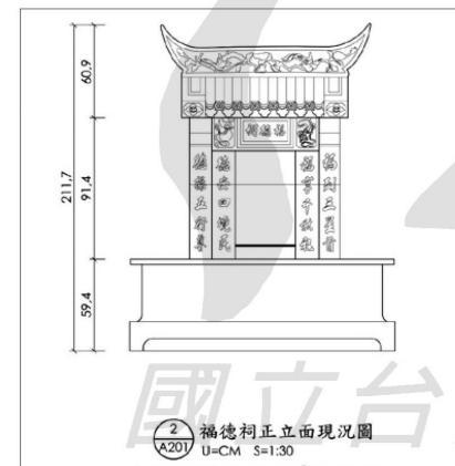
圖40 福德祠正立面現況圖，圖片來源：陳華興繪製，《縣定古蹟竹東曉江亭修復及再利用計畫》，新竹縣文化局委託，承熙建築師事務所執行，2020.5，頁3-44。
