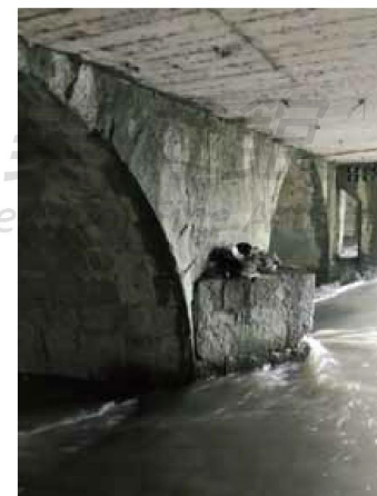
圖29 東寧橋橋墩基座三角形分水尖作法，圖片來源：吳瑞真提供（2017.3.18拍攝）。
