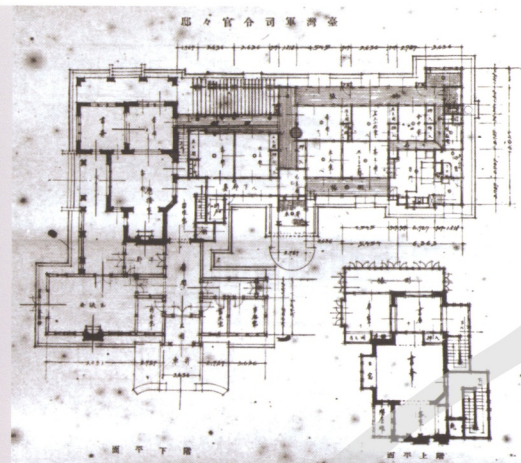
圖23 台灣軍司令官邸改築後階下平面與階上平面圖（採自《台灣建築會誌》2輯1號）
