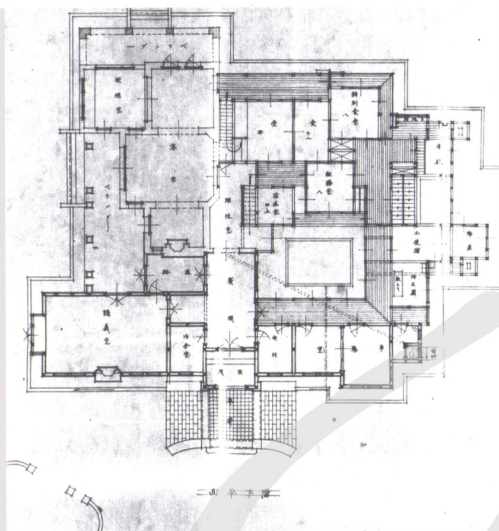
圖19 台灣軍司令官宿舍在來階下平面圖 (採自《台灣總督府公文類纂》11277卷)
