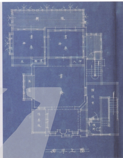
圖20 台灣軍司令官宿舍在來階上平面圖 (採自《台灣總督府公文類纂》11277卷)
