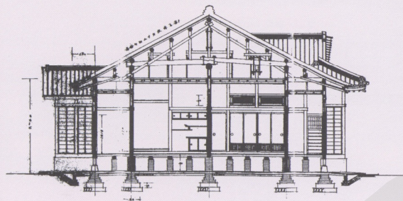
圖27 台灣軍司令官官邸改築工事斷面圖（採自《台灣總督府公文類纂》11277卷）
